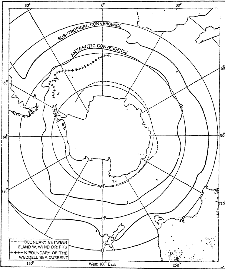
चित्र ७२—एंटार्कटिक और उपउष्णकटिबंधीय अभिविन्दुताएँ (After Deacon).
